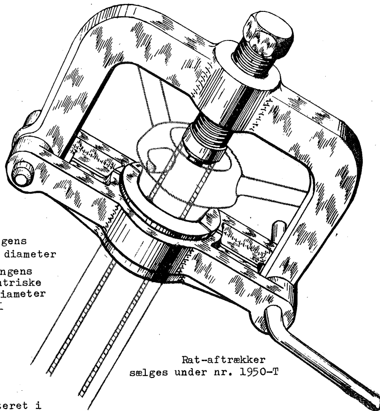
Fig. 2. Afmontering af rattet
