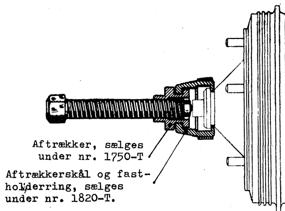
Fig. 1 - Aftrækning af nav
