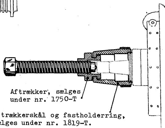
Fig. 2 - Aftrækning af kugleleje
