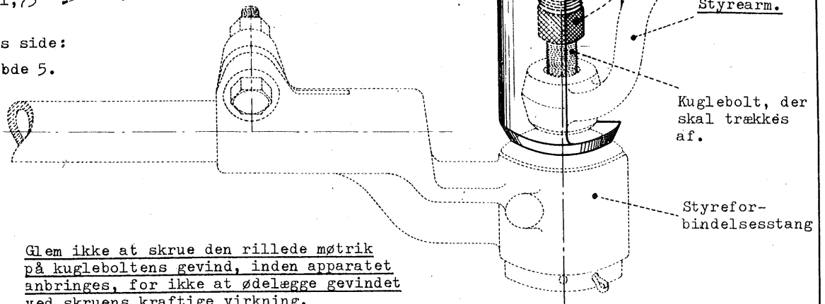
Fig. 2. Anvendelse af kuglebolt-aftrækkeren.
