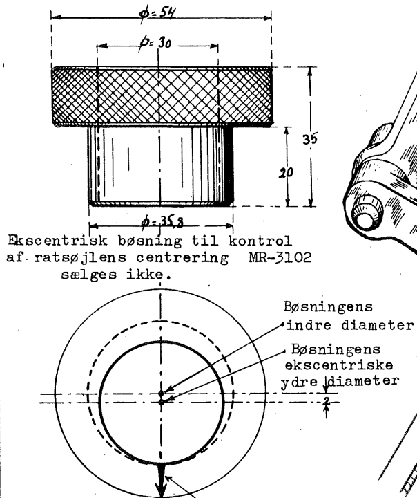
Fig. 1. Centrering af ratsøjlen
